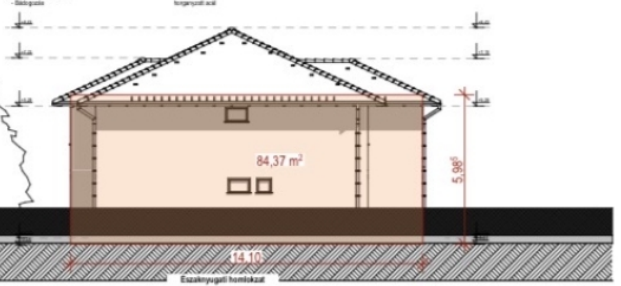
Északnyugati homlokzat
